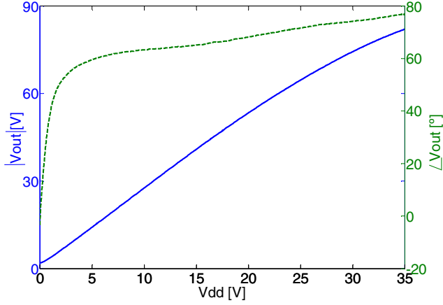
Fig. 5. (-) V_{dd} -to-AM and (--) V_{dd} -to-PM profiles.
